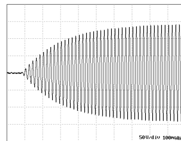
出力 ON 立ち上がり波形
