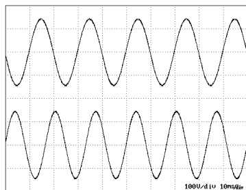
上：50Hz 出力波形 下：60Hz 出力波形
