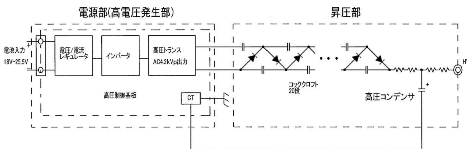
80kV 直流高圧電源 回路ブロック図
