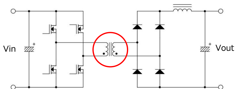
絶縁型 DC/DC コンバータ回路
