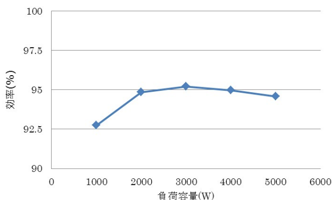
効率特性 (GL0070, エージング 1h 後)
